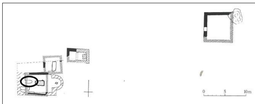
Tav. 5. 1. Ossuccio, chiesa di S. Sisinnio e S. Agata (n. 14). 2-3. Garlate, chiesa di S. Stefano (n. 17). A sinistra la planimetria del mausoleo funerario; a destra la planimetria del sacello funerario. 4. Corces, chiesa di S. Giorgio (n. 26) e i mausolei nelle vicinanze.
