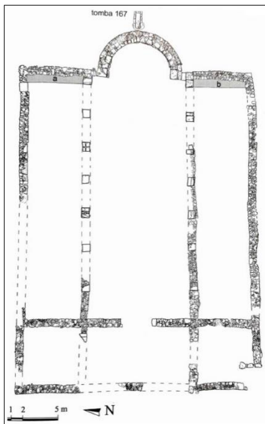
Tav. 17. 1. Rutigliano, chiesa di S. Apollinare (n. 56). (La tomba 6 è erroneamente indicata come tomba 7). 2. Vaste, fondo Giuliano, chiesa dei Santi Stefani (n. 58). 3. Torre S. Susanna, chiesa di S. Pietro a Crepacore (n. 57).
