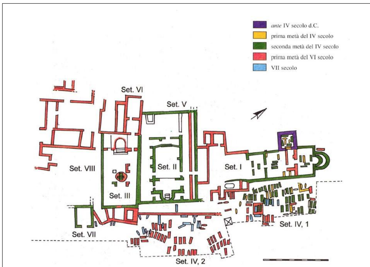
Tav. 18. 1. Sofiana (n. 60), basilica paleocristiana. 2. Cornus, complesso episcopale e area cimiteriale orientale (n. 63).
