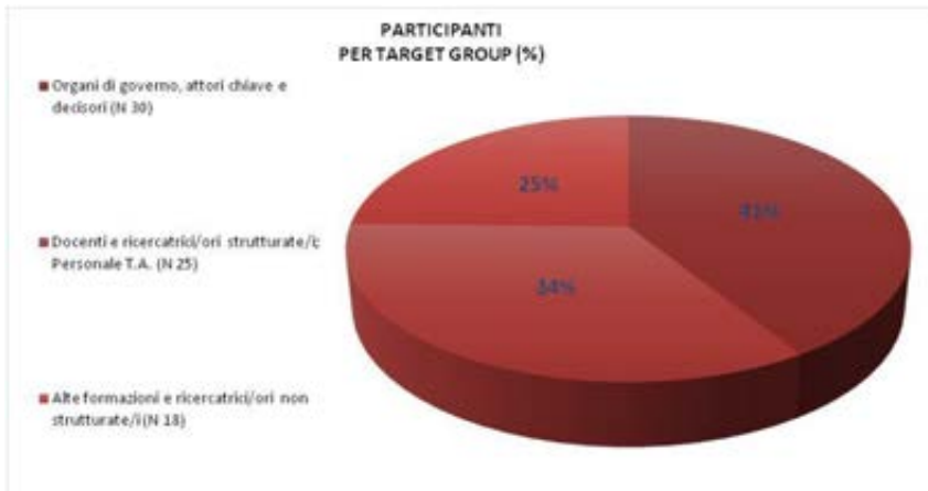
Grafico 1: Target identificati
