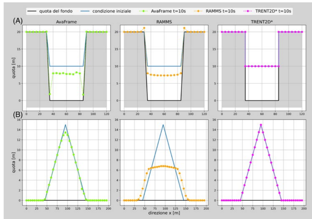
Fig. 1 - Sezione di mezzeria per: (A) test della vasca di neve ferma, (B) test della piramide di neve ferma. Linea continua: quota del fondo e della neve all'istante iniziale. Simboli: soluzione dopo 10 secondi.
