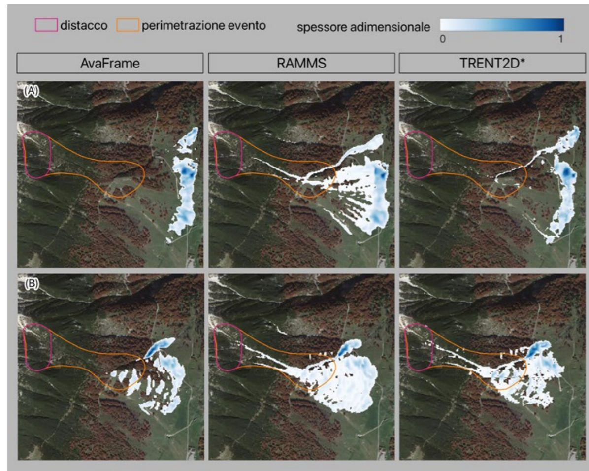
Fig. 4 - Distribuzione dell'altezza di neve adimensionalizzata per il caso della valanga di versante in zona prealpina all'istante finale della simulazione per i diversi modelli usando (A) \mu=0.22 e \xi=2500 \text{ m/s}^2 e (B) \mu=0.32 e \xi=1500 \text{ m/s}^2
