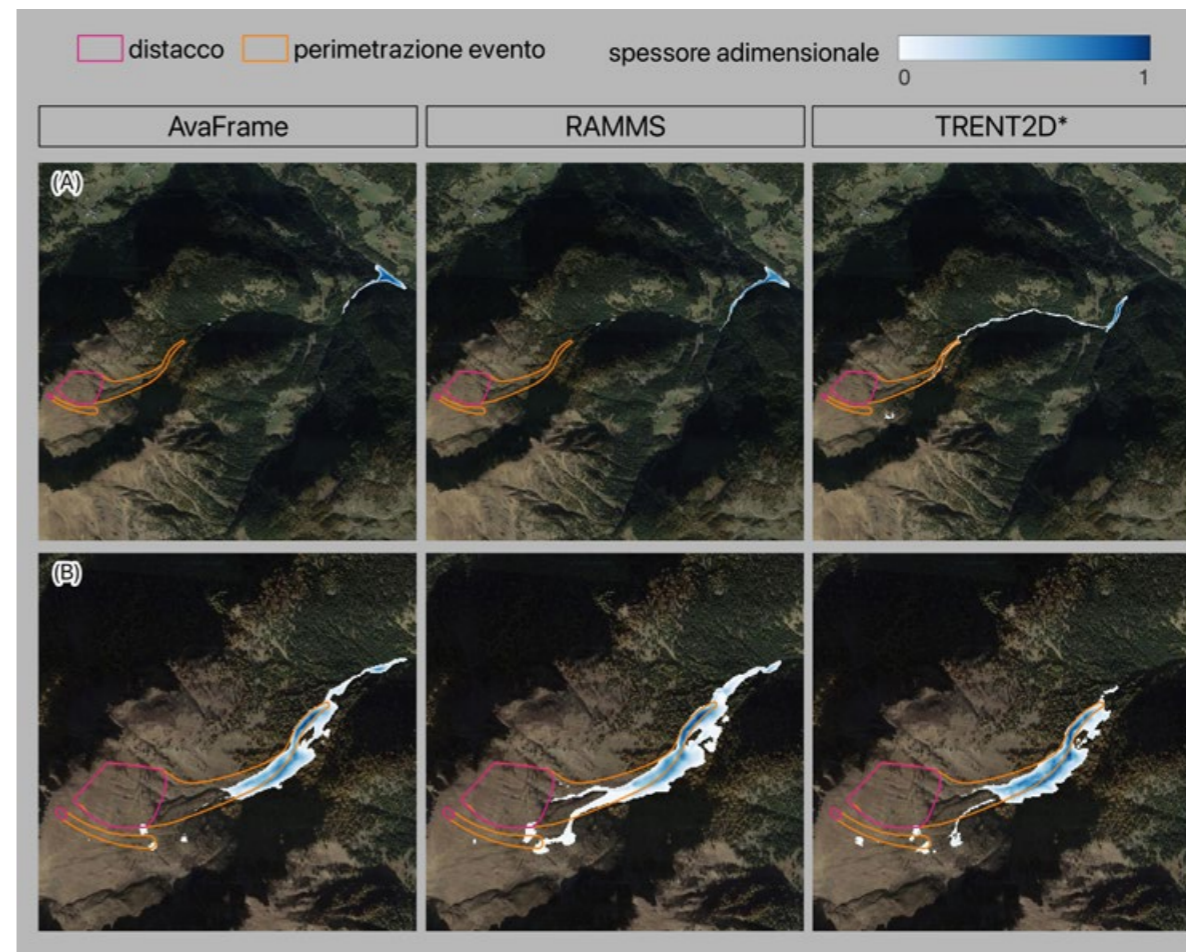
Fig. 3 - Distribuzione dell'altezza di neve adimensionalizzata per il caso della valanga di versante in zona dolomitica all'istante finale della simulazione per i diversi modelli usando (A) \mu=0.18 e \xi=3000 m/s 2 e (B) \mu=0.30 e \xi=2000 m/s 2 .
