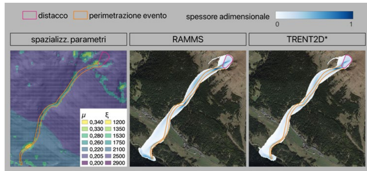
Fig. 6 - Caso della valanga incanalata in zona dolomitica. Da sinistra a destra: valore e spazializzazione dei parametri, distribuzione dell'altezza massima della neve (adimensionalizzata con il valore massimo) ottenuta dai modelli RAMMS e TRENT2D*.
