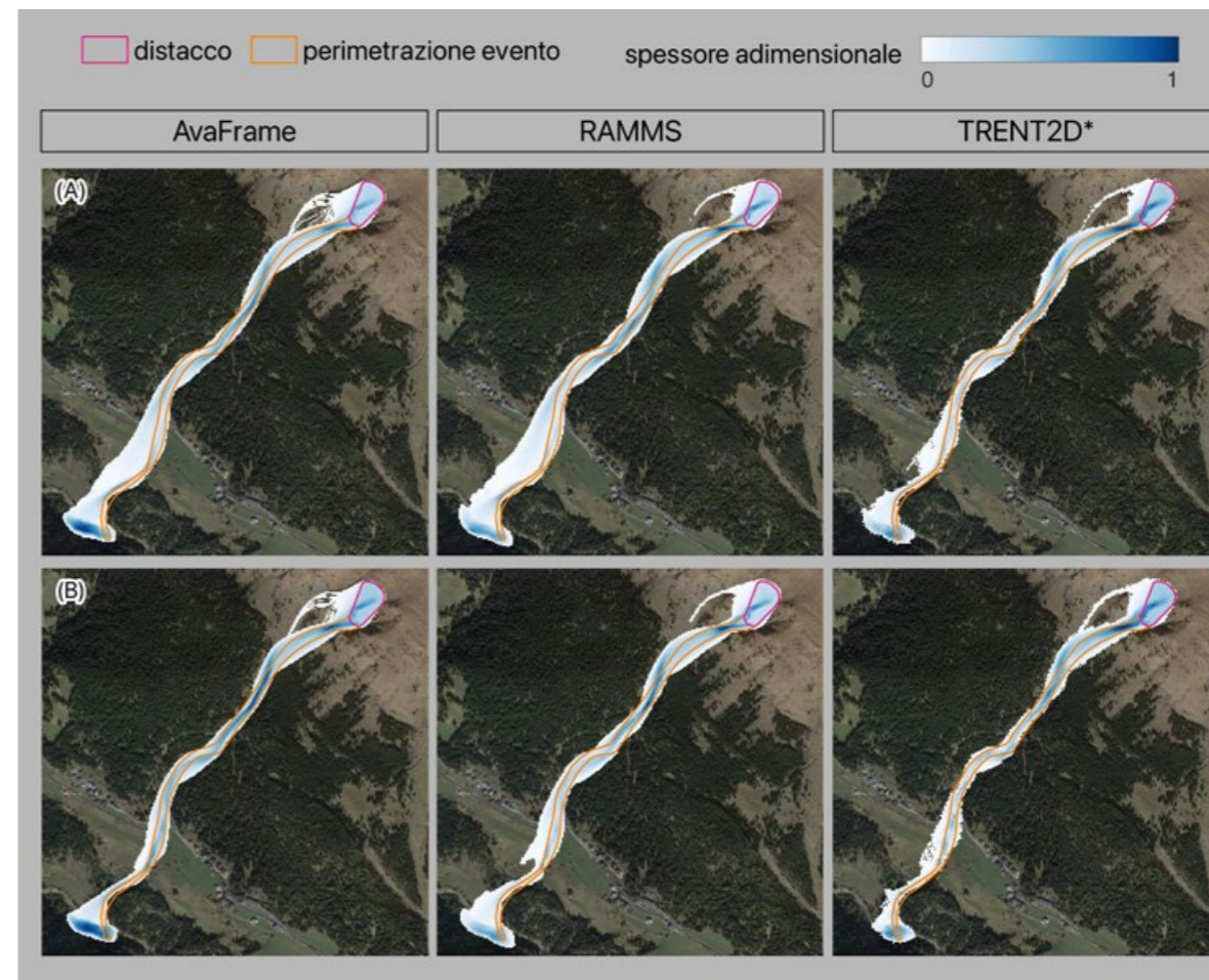
Fig. 5 - Distribuzione della massima altezza di neve adimensionalizzata per il caso della valanga incanalata in zona dolomitica all'istante finale della simulazione per i diversi modelli usando (A) \mu=0.28 e \xi=1750 \text{ m/s}^2 e (B) \mu=0.32 e \xi=1350 \text{ m/s}^2 .
