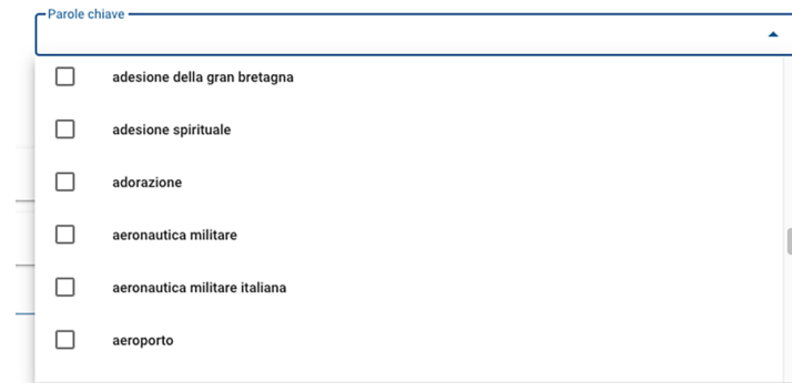
Fig. 12. Keywords filter.
