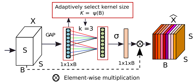
Fig. 4. EFR module.
