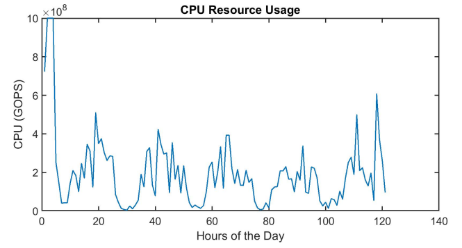
Fig. 20. Edge Data Center Resource Utilization
